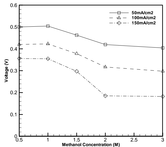
شکل (۶): تغییرات ولتاژ-غلظت متانول برای کانال با عمق ۱ میلی‌متر
