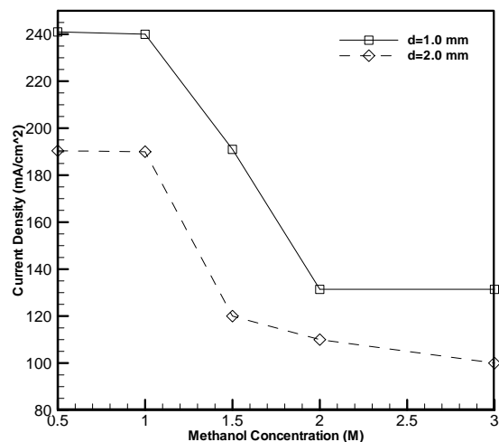
شکل (۱۱): ارتباط بین دانسیته جریان و غلظت متانول در دو عمق مختلف در ولتاژ ثابت ۰/۲۳ ولت
