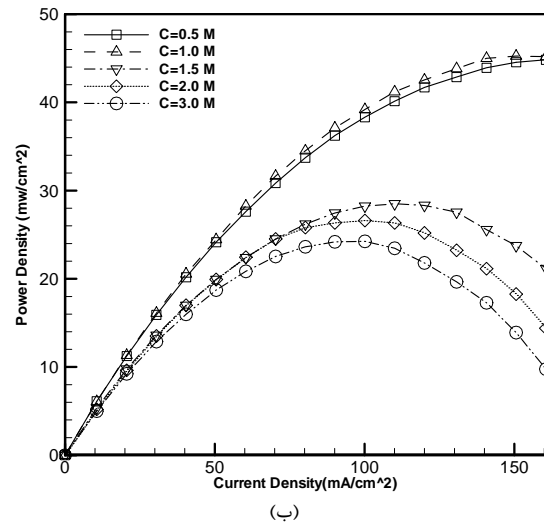
شکل (۵): (الف) نمودار تغییرات ولتاژ-دانسیتته جریان (ب) نمودار تغییرات دانسیته توان-دانسیتته جریان (عمق کانال ۲ میلی‌متر)
